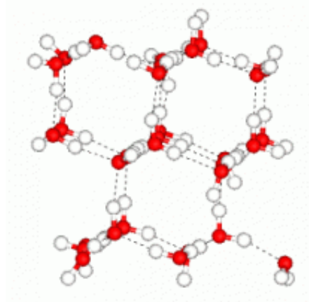
Structure cristalline hexagonale de la glace
